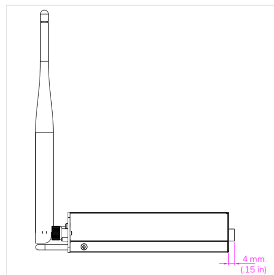
Zijaanzicht
