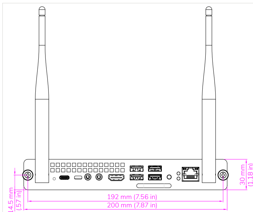
Voorraanzicht
