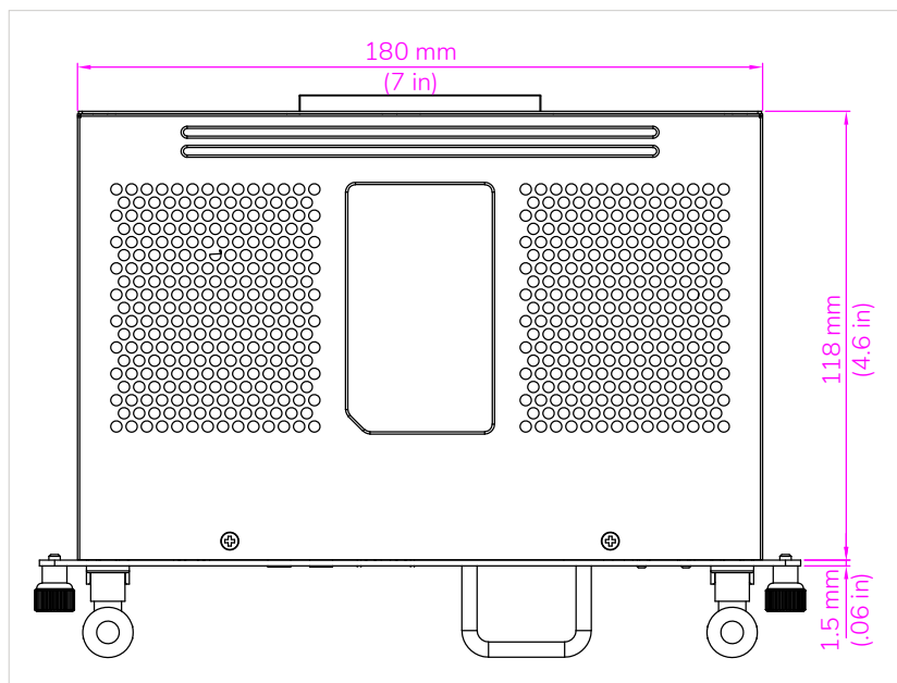
Bovenaanzicht
