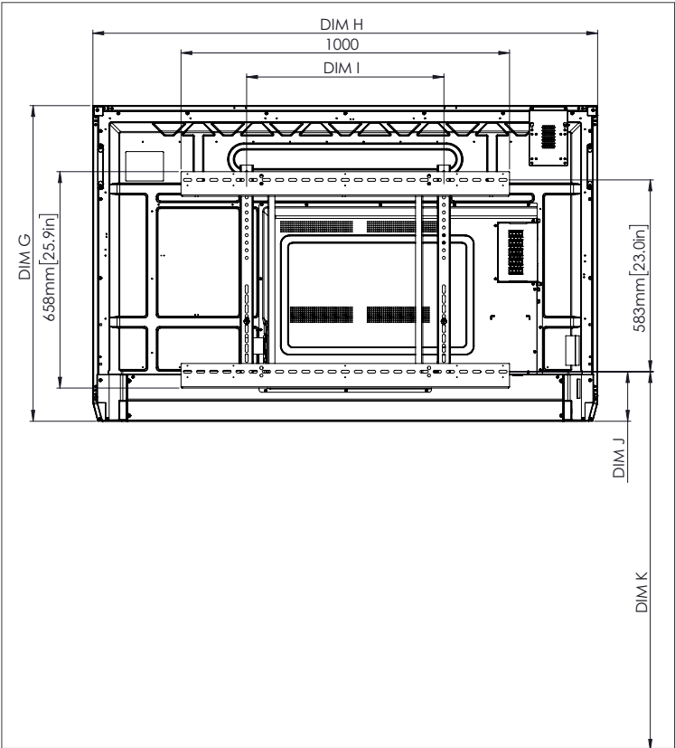
Rückan- sicht
