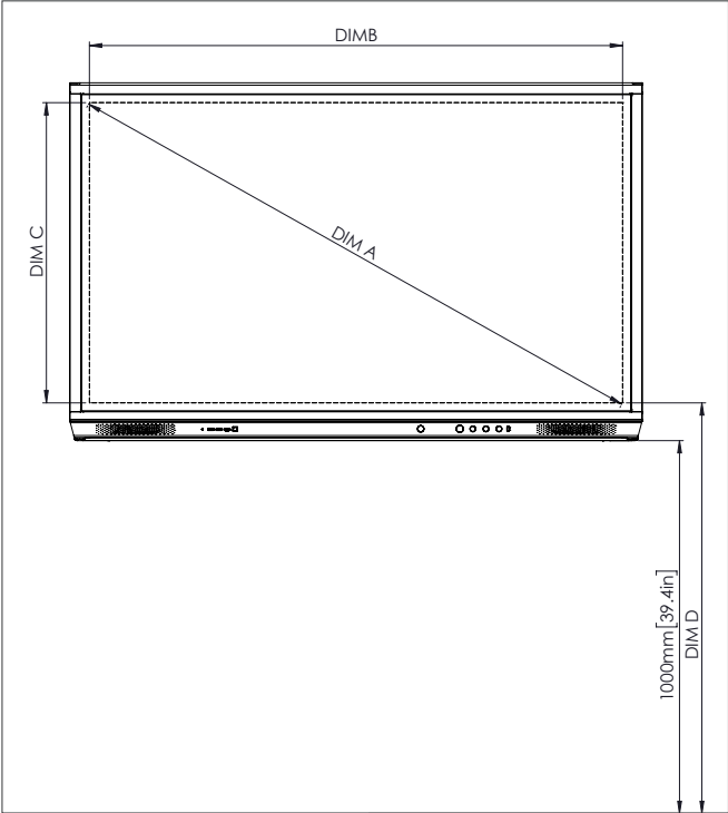
Vorder- ansicht
