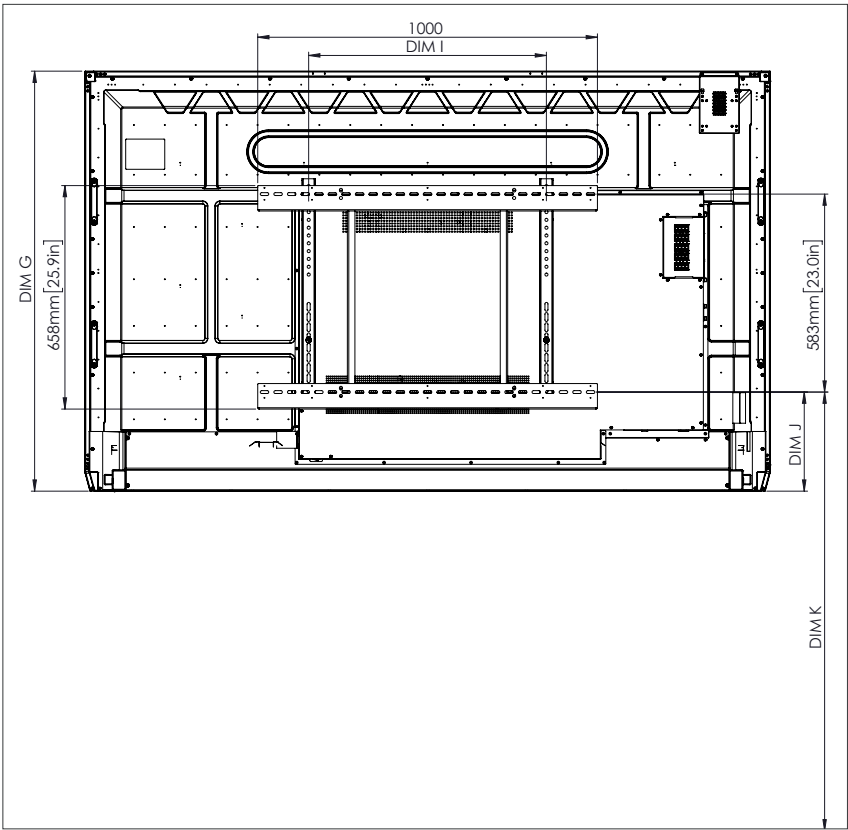
Rückansicht
