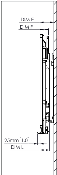
Seitenansicht
