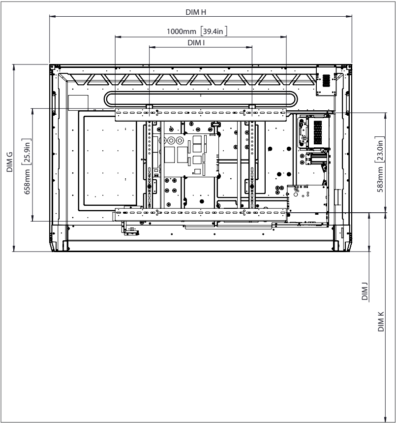
Rückansicht
